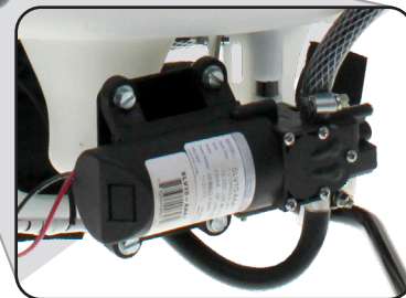
Sistema de bombeo por medio de bomba eléctrica
