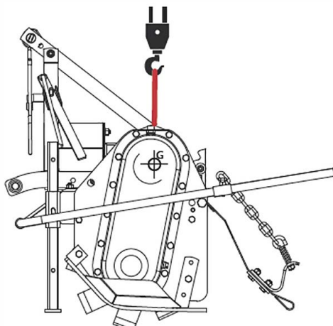
FIG. 5 Desplazamiento de la máquina
