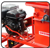
Palanca para aflojar las bandas que facilita el arranque del motor y tensarlas para su funcionamiento.
