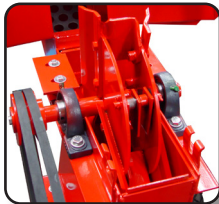
Rotor de molienda con martillos móviles y navajas volteables doble vida para moler material verde y/o seco.
