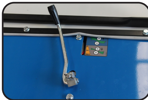
Regulador de presión de los rodillos acondicionadores
