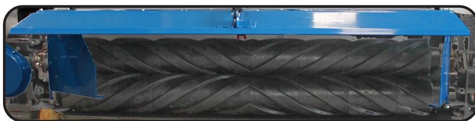
6 discos / acondicionador y dos rodillos ranurados en V
